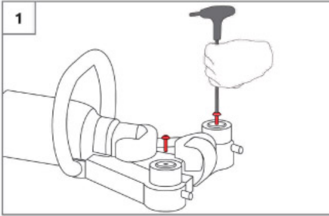
Rulmanların üzerindeki vidaları sökün
