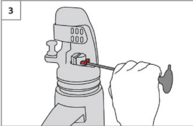
Bıçağı sabitleyin
