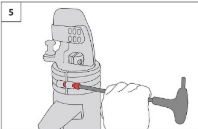
Kelepçeyi vidalayın
