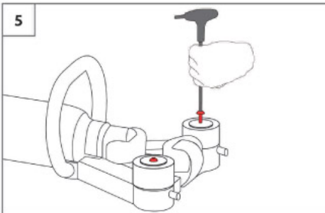
Rulmanların vidalarını sıkın
