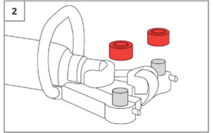
Rulmanları çıkartın
